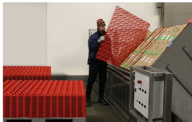
Optiflow freezer spacers vriezen niet vast aan dozen en zijn eenvoudig te ontsperen
